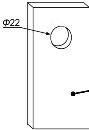
Plattjärn 160x60x10
